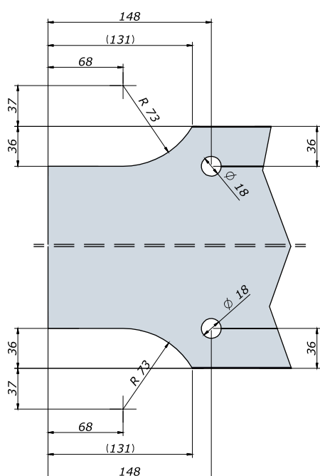
Kit cerniera idraulica incluso cerniera alta e perni di fissaggio Hydraulic hinge kit including top hinge and fixing pins
