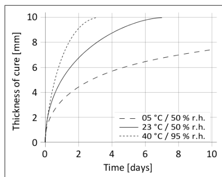
Diagram 1: Hitrost utrjevanja Sikasil® WS-605 S
